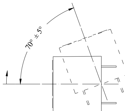
恢復動作角度: 70^\circ \pm 5^\circ restore action angle: 70^\circ \pm 5^\circ
