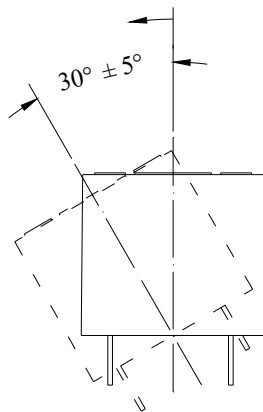
傾倒動作角度: 30^\circ \pm 5^\circ Dumping angle: 30^\circ \pm 5^\circ
