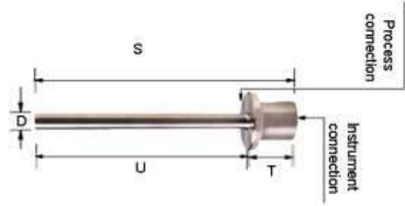
BAR STOCK VAN STONE THERMOWELL
