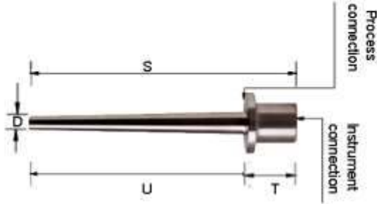
WELDED VAN STONE THERMOWELL
